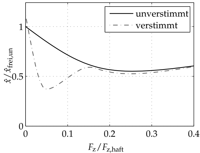
Bild 7.16: Vergleich der Dämpfungsoptimierungskurven des unverstimmten und des verstimzten Systems
