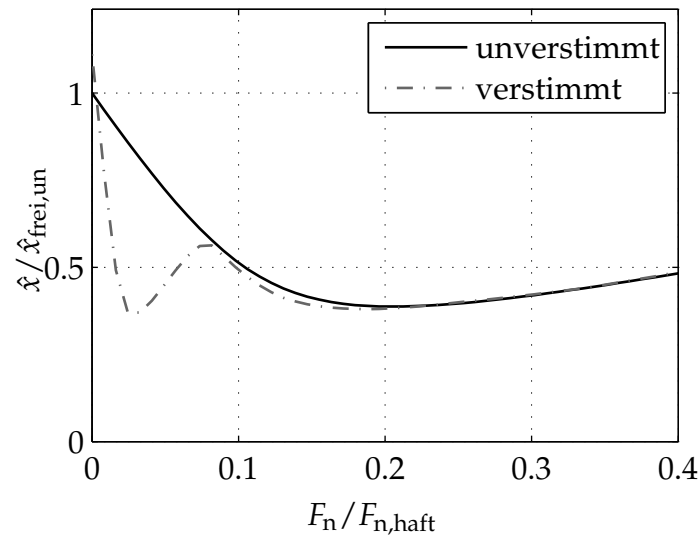
Bild 7.6: Vergleich der Dämpfungsoptimierungskurven des unverstimmten und des mit \kappa_{\text{ver}} verstimmt Systems
